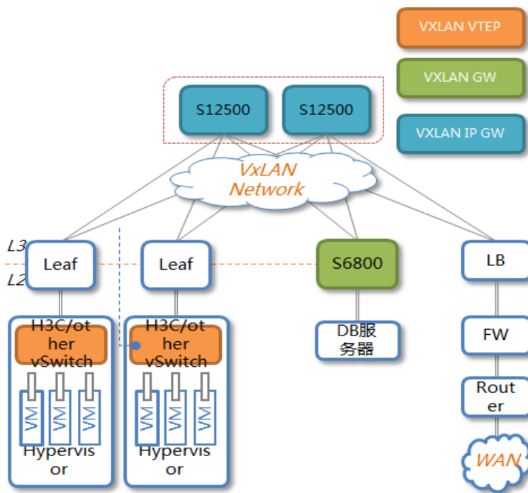
S1250 系列核心交换机 SDN/VxLAN 应用示意图
