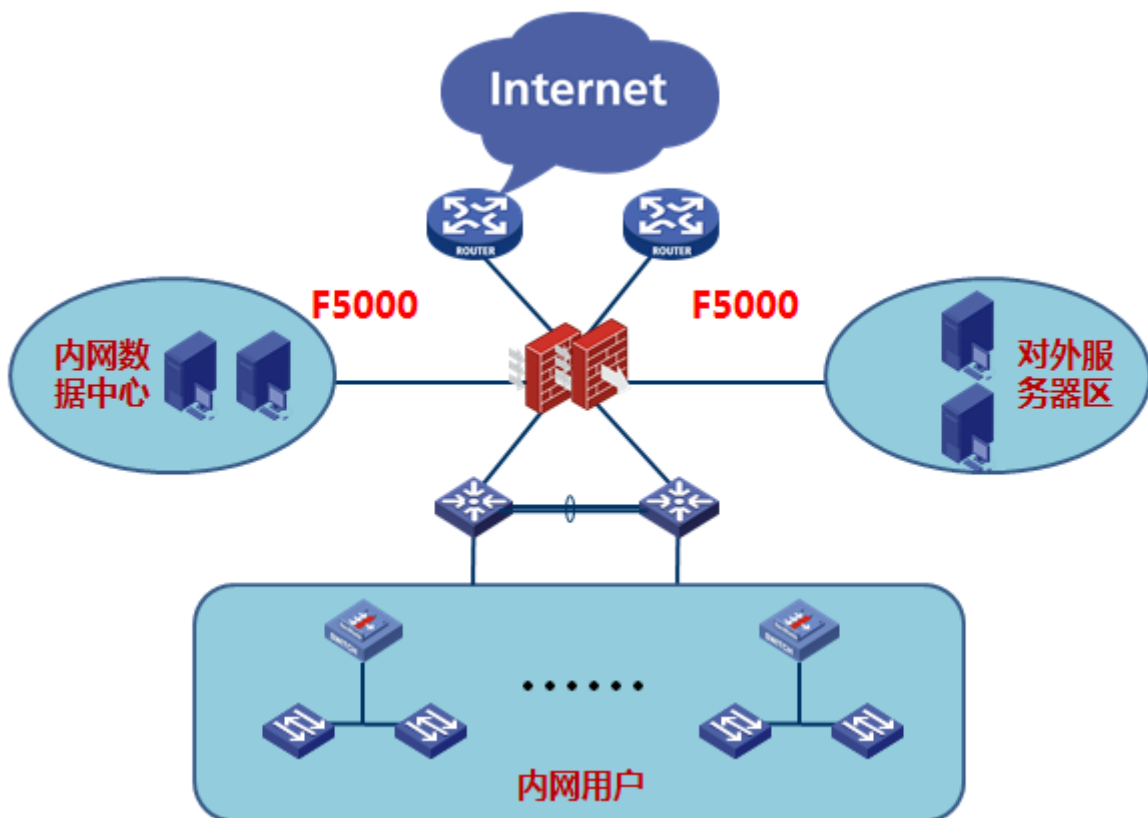
H3C SecPath F50X0 系列组网应用示意图
